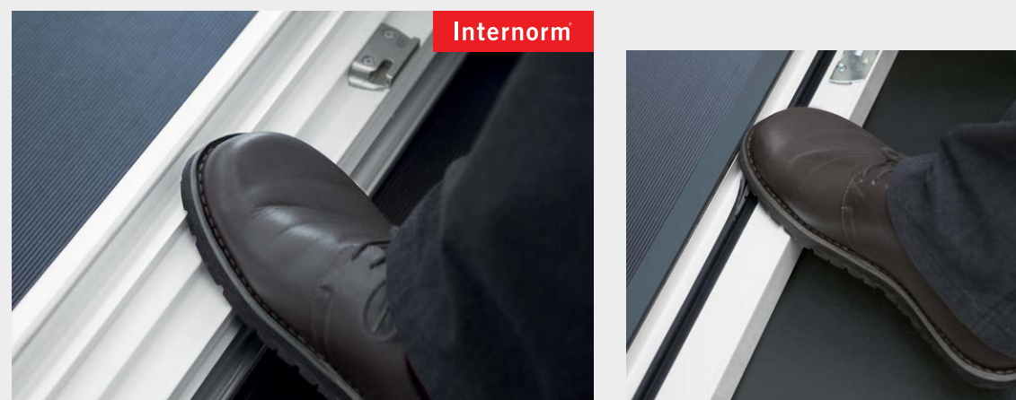
Középső tömítések az Internormnál nem a tokon, hanem a szárnyon
